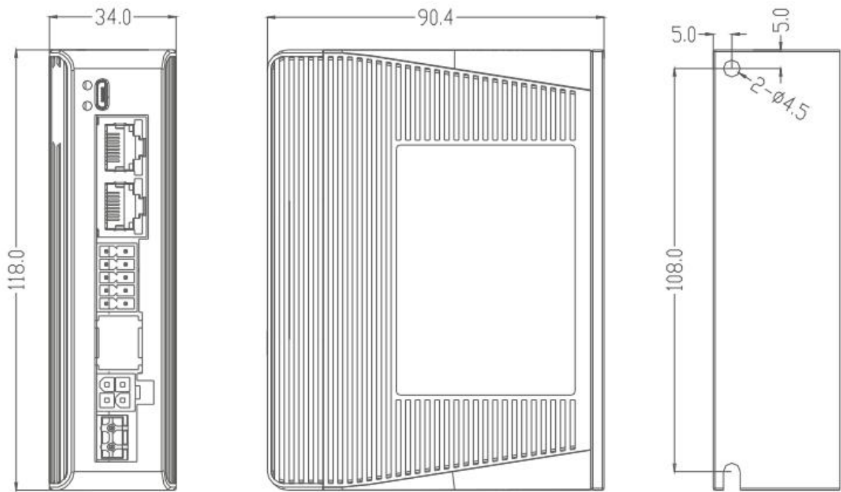
图 2-1 CL3C-EC503/507 安装尺寸图(单位：mm) ※ 设计安装尺寸时，注意考虑端子大小及布线！
