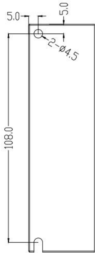
图 2-1 CL3C-EC503/CL3C-EC507 安装尺寸图(单位：mm) ※ 设计安装尺寸时，注意考虑端子大小及布线！
